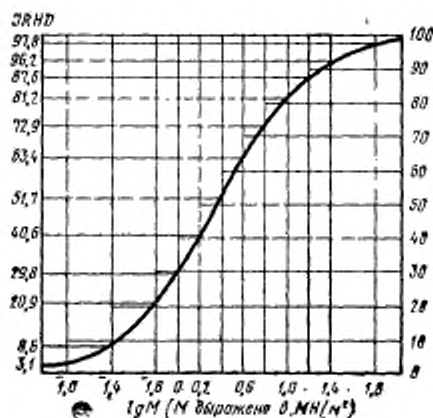
Зависимость твердости резины от модуля упругости
