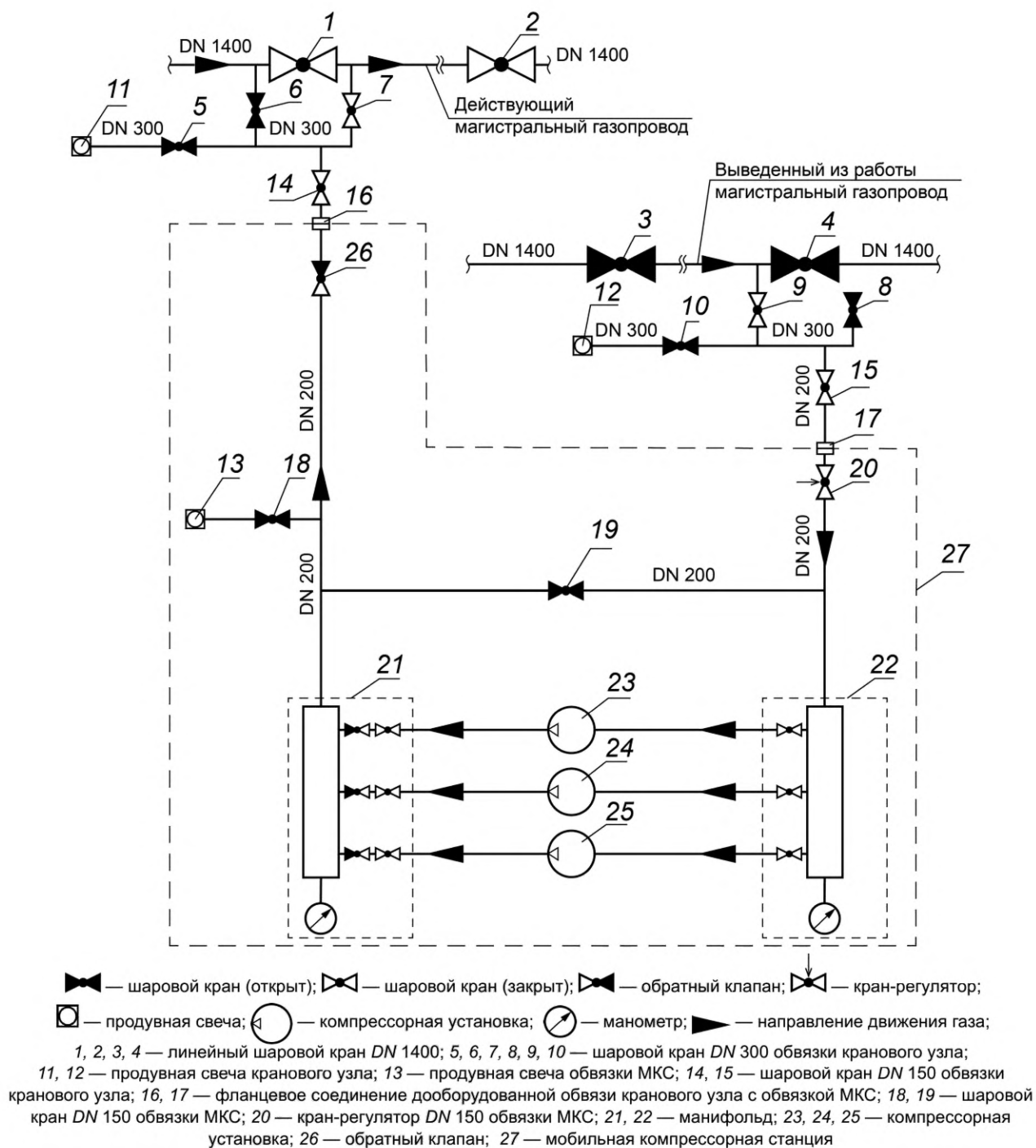
Рисунок В.1 — Типовая технологическая схема подключения мобильной компрессорной станции к магистральным газопроводам
