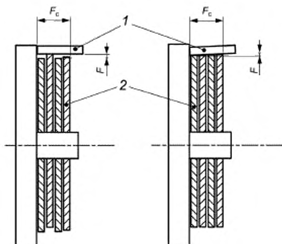
1 — стопорный элемент; 2 — комбинационные диски
