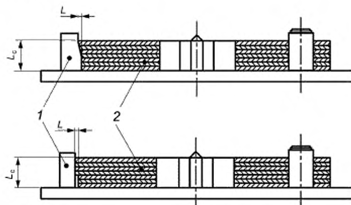
1 — стопорный элемент; 2 — сувальды
