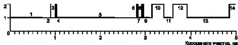
Рисунок Е.5 — Графическая иллюстрация формирования расчетных участков
