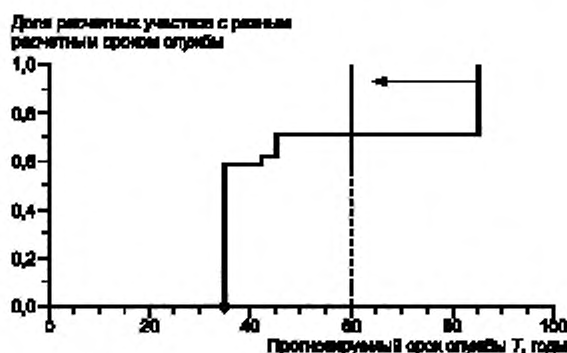
Рисунок Е.8 — Графическая иллюстрация построения кумулятивной функции распределения сроков службы расчетных участков и установления назначенного срока службы для всего участка ЛЧМГ
