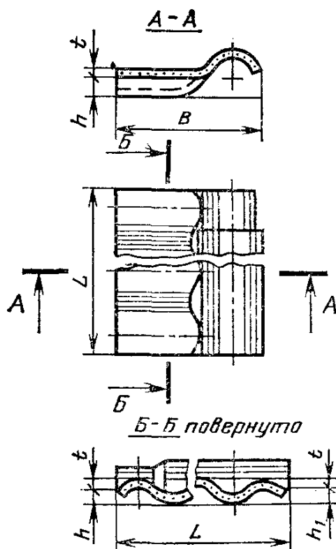
Перекрываемая деталь КС-1
