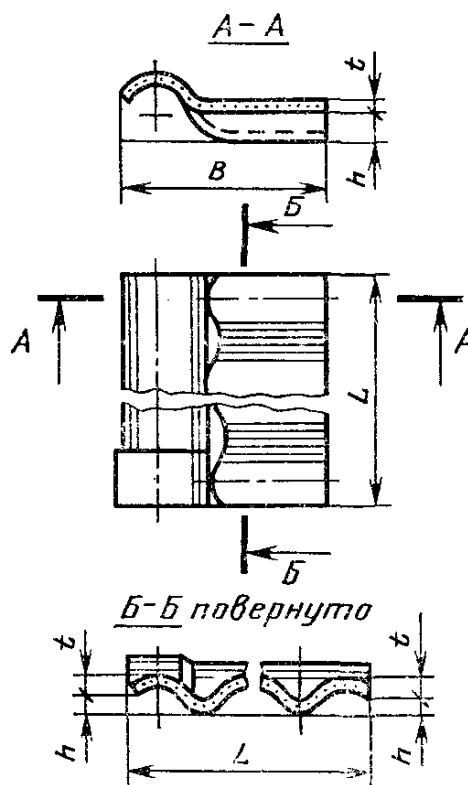
Перекрывающая деталь КС-2
