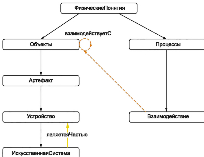
Рисунок 3 — Таксономия понятий ИскусственнаяСистема и Взаимодействие по CORAX
