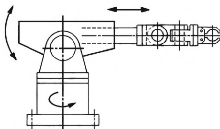
Рисунок А.3 — Робот с полярной или сферической системой координат
