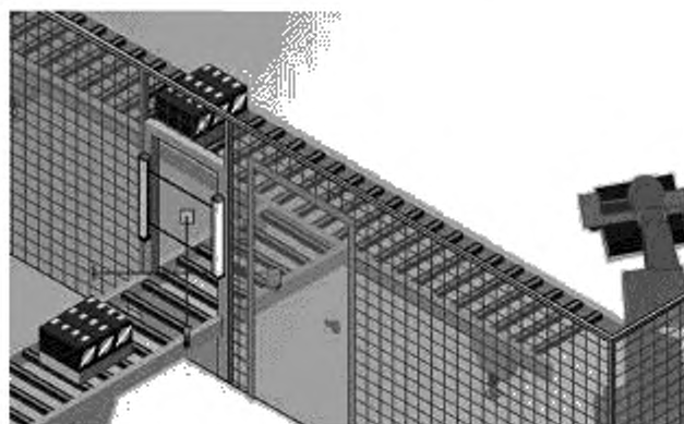
Рисунок С.4 — Обеспечение безопасности с помощью ЭЧЗО
