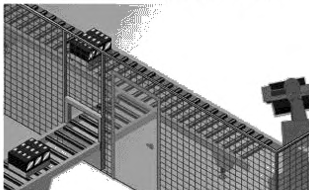
Рисунок С.2 — Подача материальных объектов через небольшое окно доступа в ограждении
