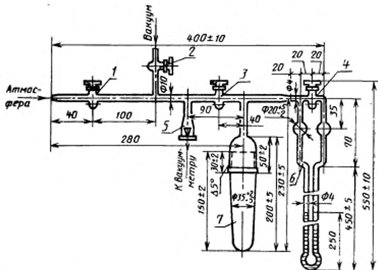
Прибор для вакуумного метода анализа (метод 2)
