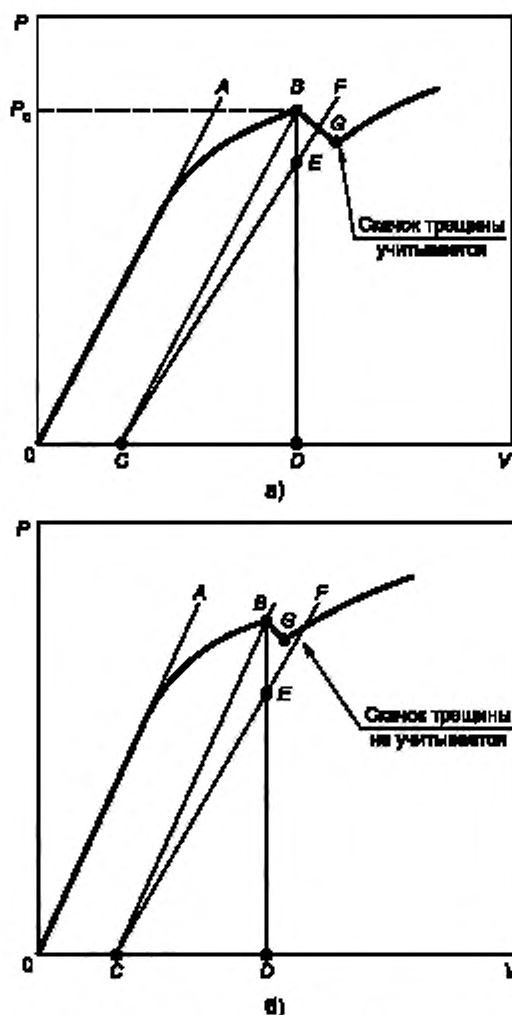
Рисунок Е.7 — Процедура оценки значимости скачка трещины
