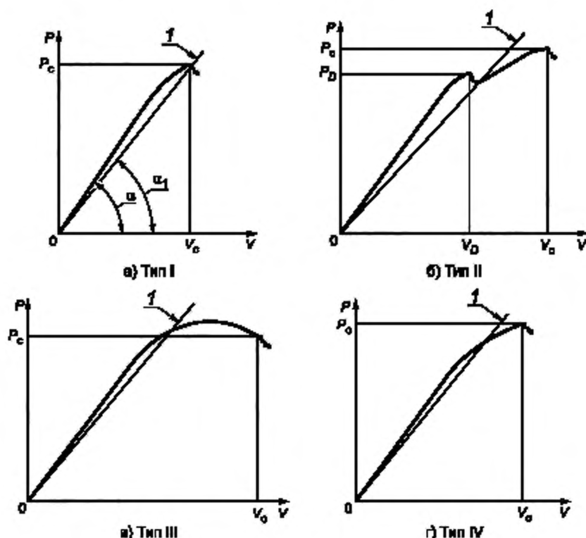
1 — 5 %-ная секущая. \tan \alpha_1 = 0,95 \tan \alpha ; P_c — нагрузка при разрушении образца; P_D — нагрузка локального максимума
