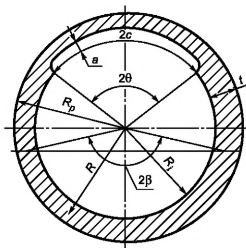
Рисунок А.2 — Труба с окружной трещиной
