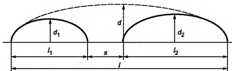
Рисунок А.3 — Объединение дефектов при коррозионном растрескивании
