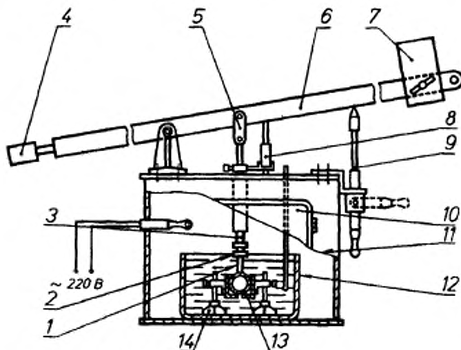
1 — стержень; 2 — гайка; 3 — опора; 4 — верньер; 5 — серьга; 6 — рычажное устройство; 7 — груз; 8 — индикатор; 9 — регулирующий упор; 10 — стеклянная дверь; 11 — металлический корпус; 12 — резервуар; 13 — испытываемая деталь; 14 — фиксирующее приспособление
