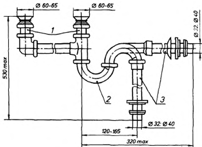
1 — выпуск; 2 — корпус сифона, 3 — отвод
