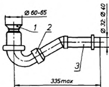
1 — выпуск; 2 — корпус сифона; 3 — отвод
