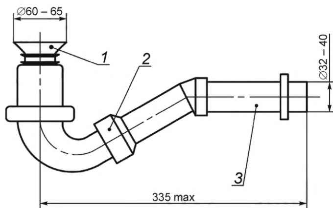
1 — выпуск; 2 — корпус сифона; 3 — отвод
