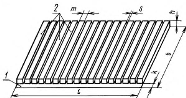
1 — покрывной материал; 2 — минераловатные полосы
