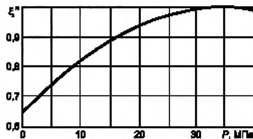
Рисунок 8 — Поправочные коэффициенты \xi' и \xi''
