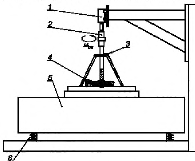
1 — электродвигатель; 2 — вибратор; 3 — ограничивающее устройство, 4 — опытный объект 5 — станина стенов; 6 — пружины
