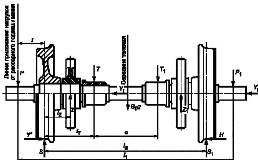
Рисунки А.1 и А.2: T(T_1) — вертикальная сила от опорно-осевого подшипника, P(P_1) — вертикальная нагрузка на буксовую шейку оси со стороны набегавшего (сбегавшего) колеса, S(S_1) — вертикальная нагрузка на набегавшее (сбегавшее) колесо от рельса; Z(Z_1) — вертикальная сила на ось от ведомой шестерни; H — поперечная составляющая силы трения внутреннего колеса о рельс; Y — боковая сила рельса на набегавшее колесо; Y_1 — поперечная сила инерции КП; Y_p — рамная сила; l — расстояние от середины буксовой шейки до плоскости круга катания соседнего колеса; l_1 — расстояние между линиями приложения вертикальной нагрузки к буксовым шейкам оси КП; l_2 — расстояние между плоскостями кругов катания КП; l_3 — расстояние от плоскости круга катания набегавшего колеса до линии действия силы T ; l_4 — расстояние от плоскости круга катания набегавшего колеса до линии действия силы Z ; G_0g — масса части оси, заключенной между плоскостями кругов катания колес; g — ускорение силы тяжести. a — расстояние между силами T и T_1 ; a_1 — расстояние от середины тележки до силы T_1 ; a_2 — расстояние между силами T и Z .
