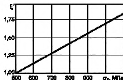
Рисунок 7 — Поправочные коэффициенты \xi' и \xi''
