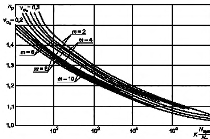
Рисунок 9 — Диаграмма для определения n_p
