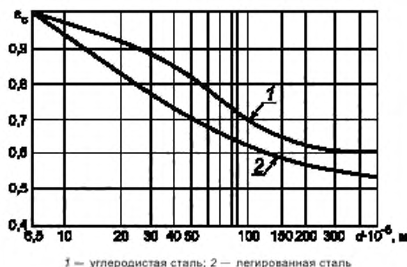
Рисунок 4 — Коэффициенты влияния абсолютных размеров сечения k на усталостную прочность
