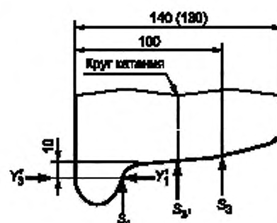
S , \gamma — вертикальная и боковая нагрузки на набегавшее колесо от рельса при режимах: S_1 — движение по кривым участкам пути; S_2 — движение высокоскоростного ПС по специальному пути, S_3 — движение по стрелкам
