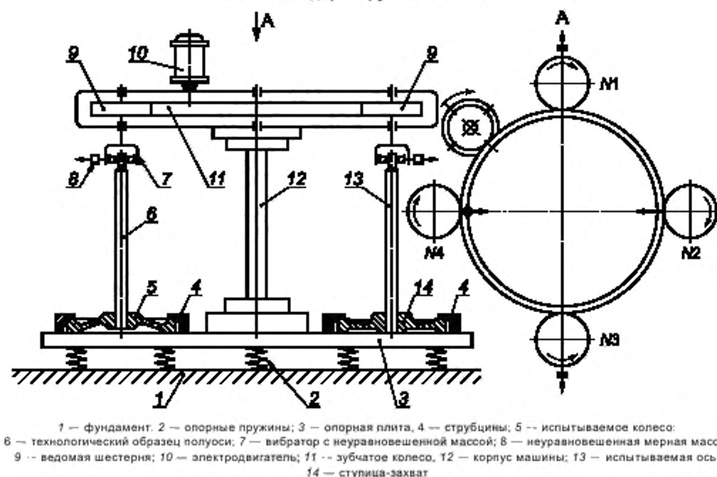
Рисунок Ж.1 — Пример схемы стенов для испытания на усталость колес и осей
