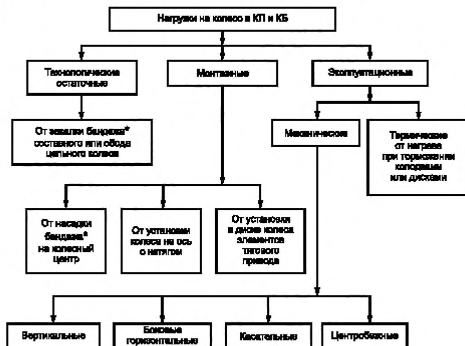
Рисунок 1 – Виды нагрузок, действующих на колесо
