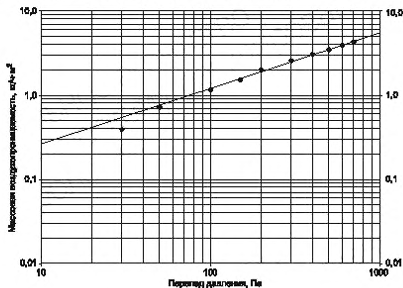
Рисунок Б.1 — Пример графика зависимости массовой воздухопроницаемости q_v от перепада давления \Delta P
