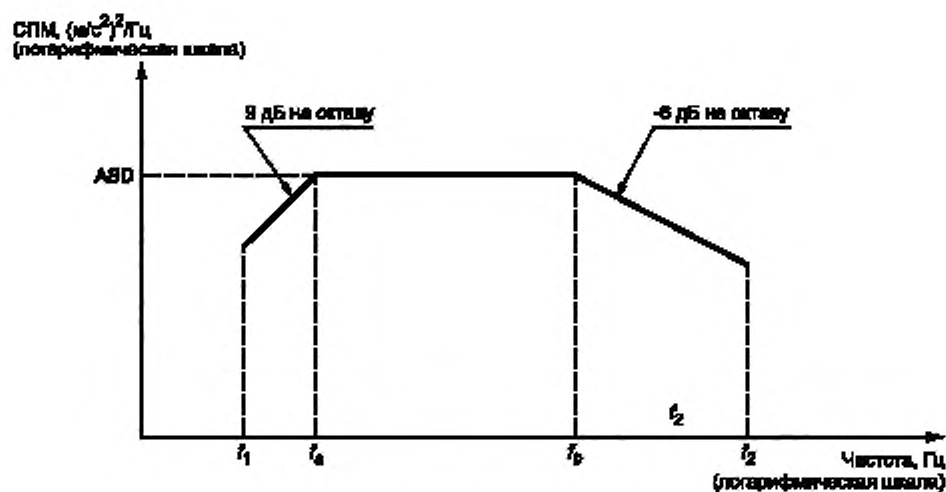
Рисунок С.1 — СПМ виброускорений
