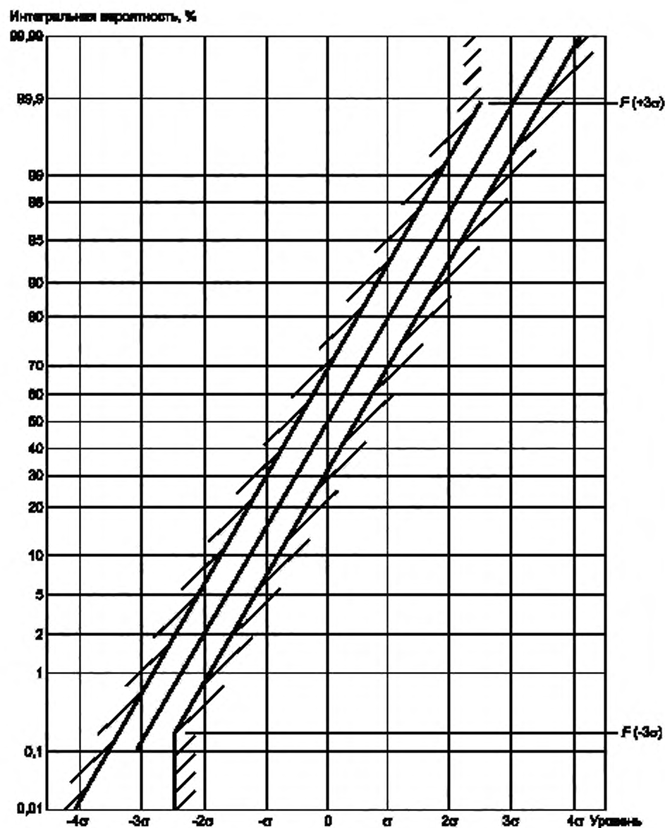
Рисунок 6 — Поля допуска для интегральной плотности распределения вероятности
