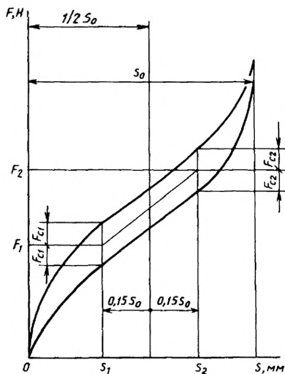
Рисунок 2 — Упругая характеристика сиденья
