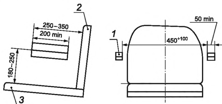
1 — подлокотник; 2, 3 — подушки сиденья
