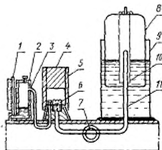
1—манометр; 2—резервуар; 3—соединительная трубка; 4—образец; 5—гильза; 6—вилка; 7—трехходовой кран; 8—колокол; 9—бак; 10—трубка колокола; 11—трубка бака
