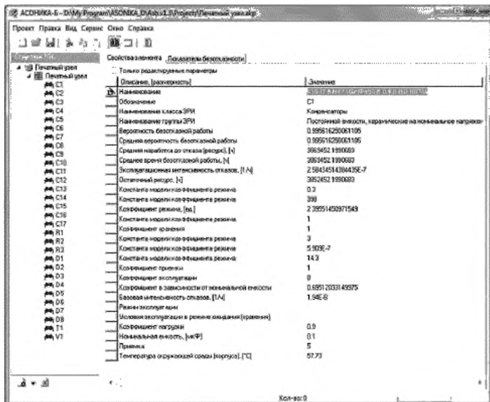
Рисунок Б.6 — Анализ показателей надежности в подсистеме АСОНИКА-Б: задание исходных данных
