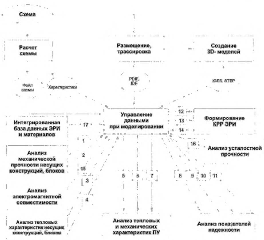
Рисунок 4.1 — Структура комплексной модели надежности БЗ РТК на основе сквозного автоматизированного моделирования физических процессов
