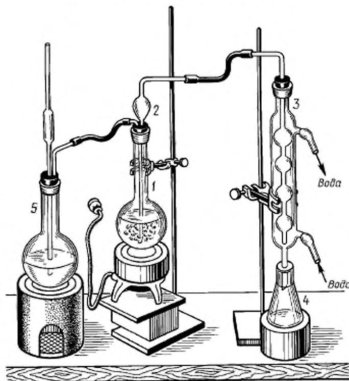
Прибор для отгонки летучих жирных кислот
