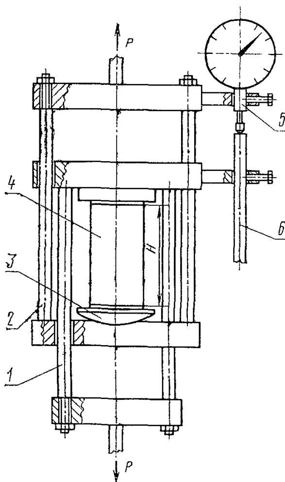
1 — нижняя траверса реверсора; 2 — верхняя траверса реверсора; 3 — шарнирная опора, 4 — образец; 5 — индикатор; 6 — упорный шток.
