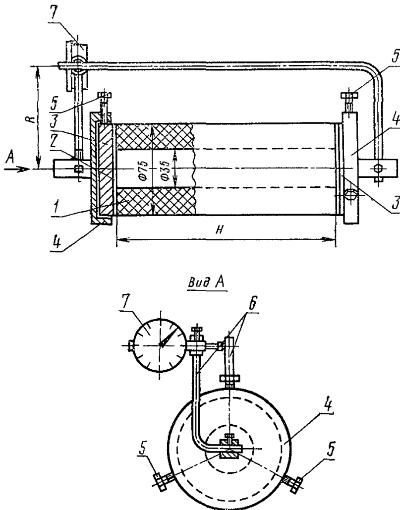
Образец и приспособление для определения модуля сдвига
