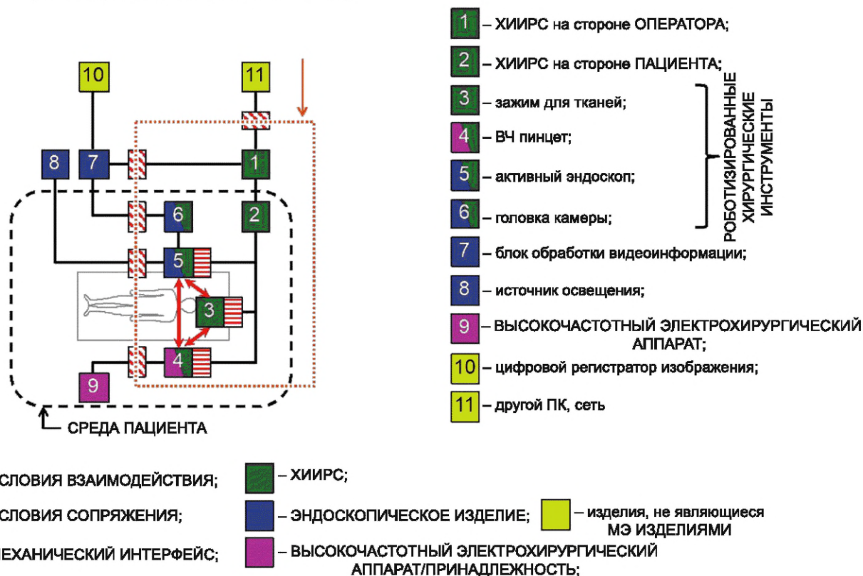
Рисунок 201.АА.102 — Пример КОНФИГУРАЦИИ ОБОРУДОВАНИЯ, ИСПОЛЬЗУЮЩЕГО СРЕДСТВА РОБОТОТЕХНИКИ для лапароскопии
