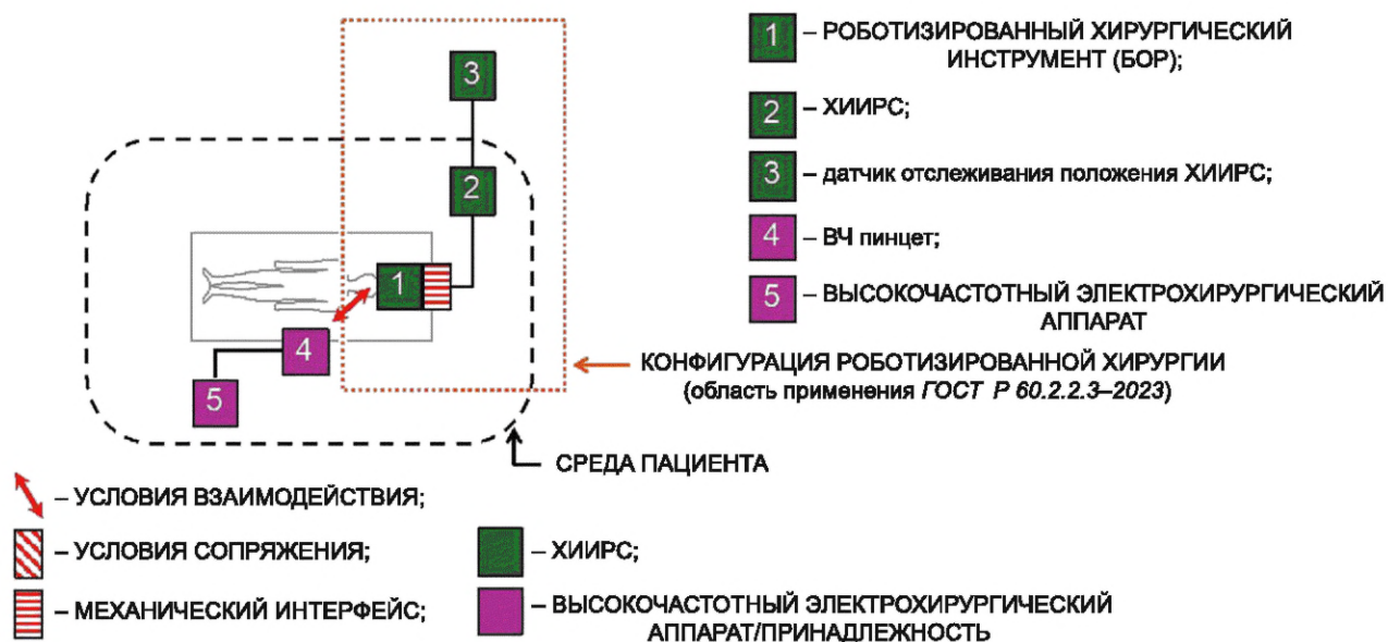
Рисунок 201.АА.103 — Пример КОНФИГУРАЦИИ ОБОРУДОВАНИЯ, ИСПОЛЬЗУЮЩЕГО СРЕДСТВА РОБОТОТЕХНИКИ, для сверления костей
