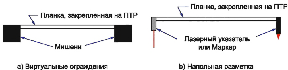
Рисунок 13 — Расположенное на ПТР оборудование для испытаний
