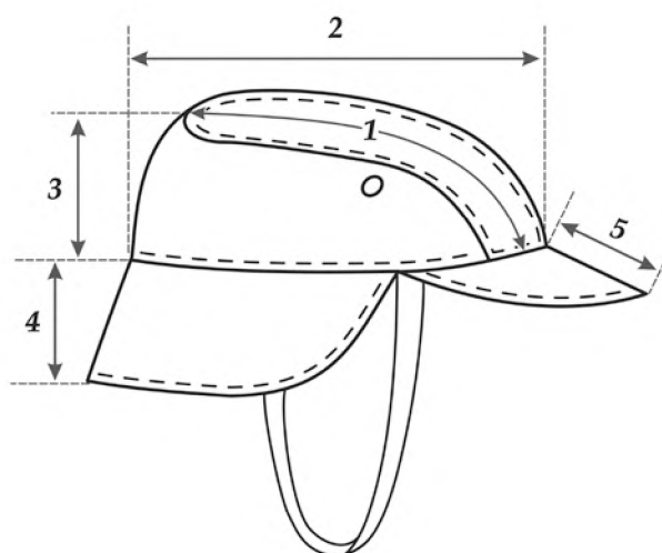
Рисунок 3 – Места измерений головного убора мужского летного
