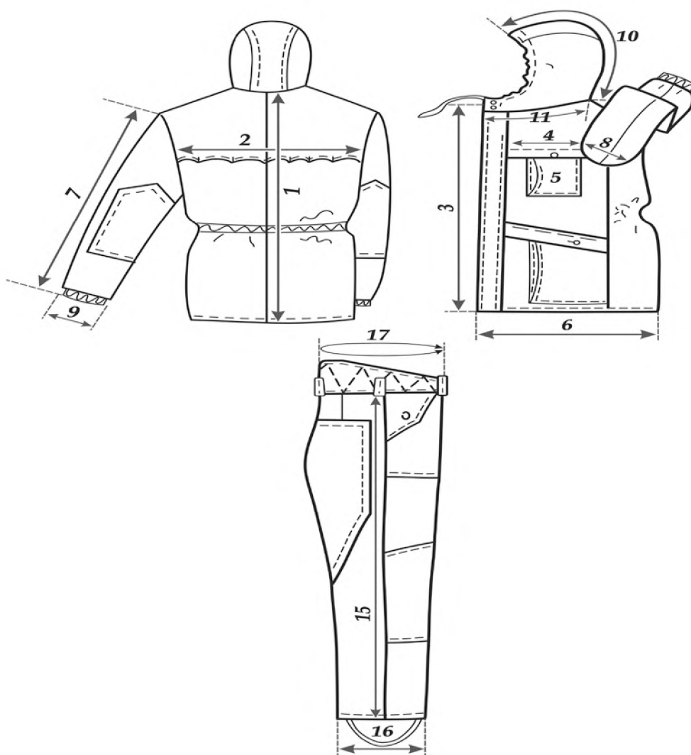
Рисунок 2 – Места измерений костюма мужского летного
