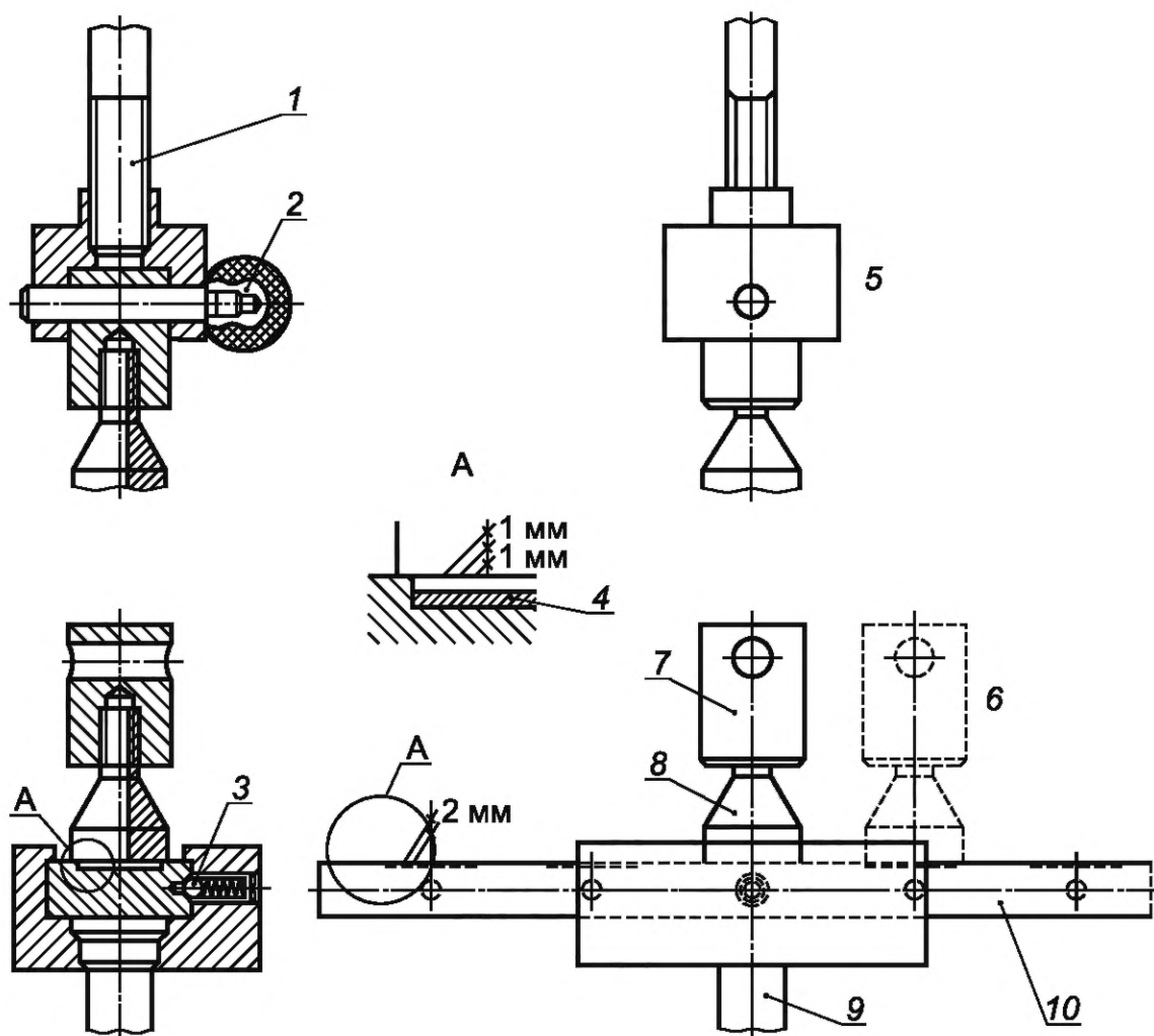
1 — тяга (захват установки для испытаний с универсальным шарниром); 2 — крепление штифта шарнира; 3 — подпружиненный стопор в ползунковом кондукторе; 4 — эпоксидная смола; 5 — тяга с универсальным шарниром; 6 — тяга с универсальным шарниром (общий вид верхней части устройства); 7 — универсальный шарнир; 8 — конический штамп с хвостовиком; 9 — тяга (захват) установки для испытаний; 10 — модульная рейка с цилиндрическими углублениями
