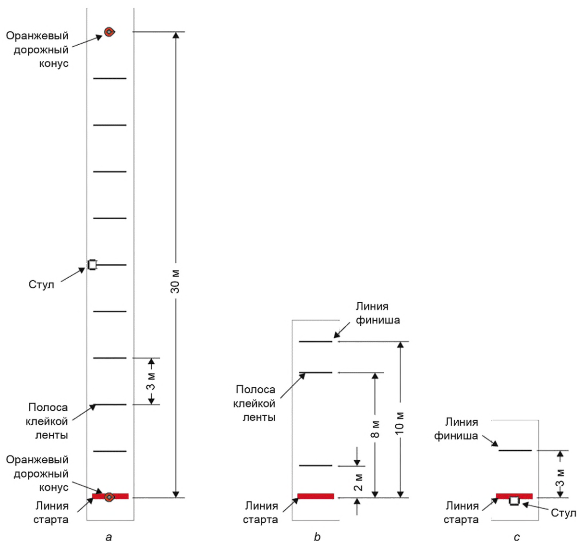
а — испытание 6МХ; б — испытание 10МХ; в — испытание ВП
