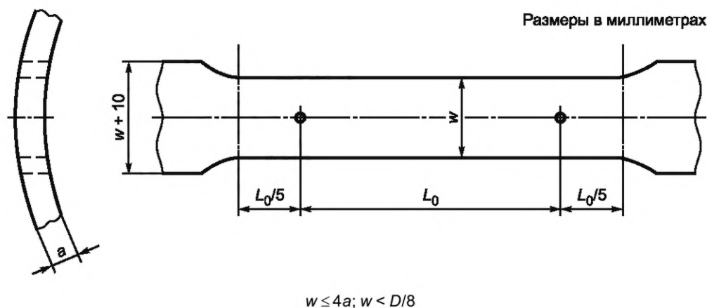
Рисунок 6 — Образец для испытания на растяжение
