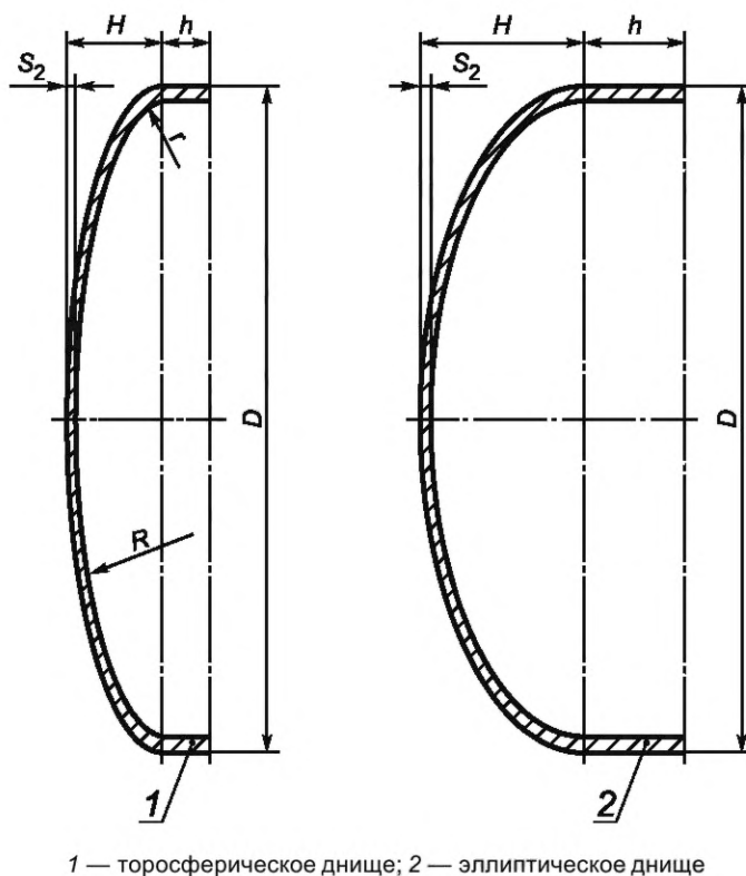
Рисунок 1 — Иллюстрация конструкций днищ, разрешенных к использованию
