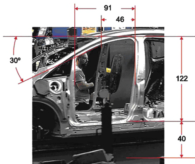
a — пример реального проема под дверь автомобиля
