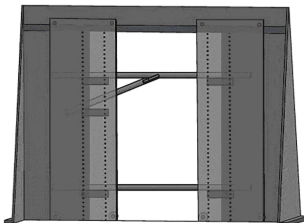
b — конструкция испытательного оборудования, имитирующая проем под дверь автомобиля
