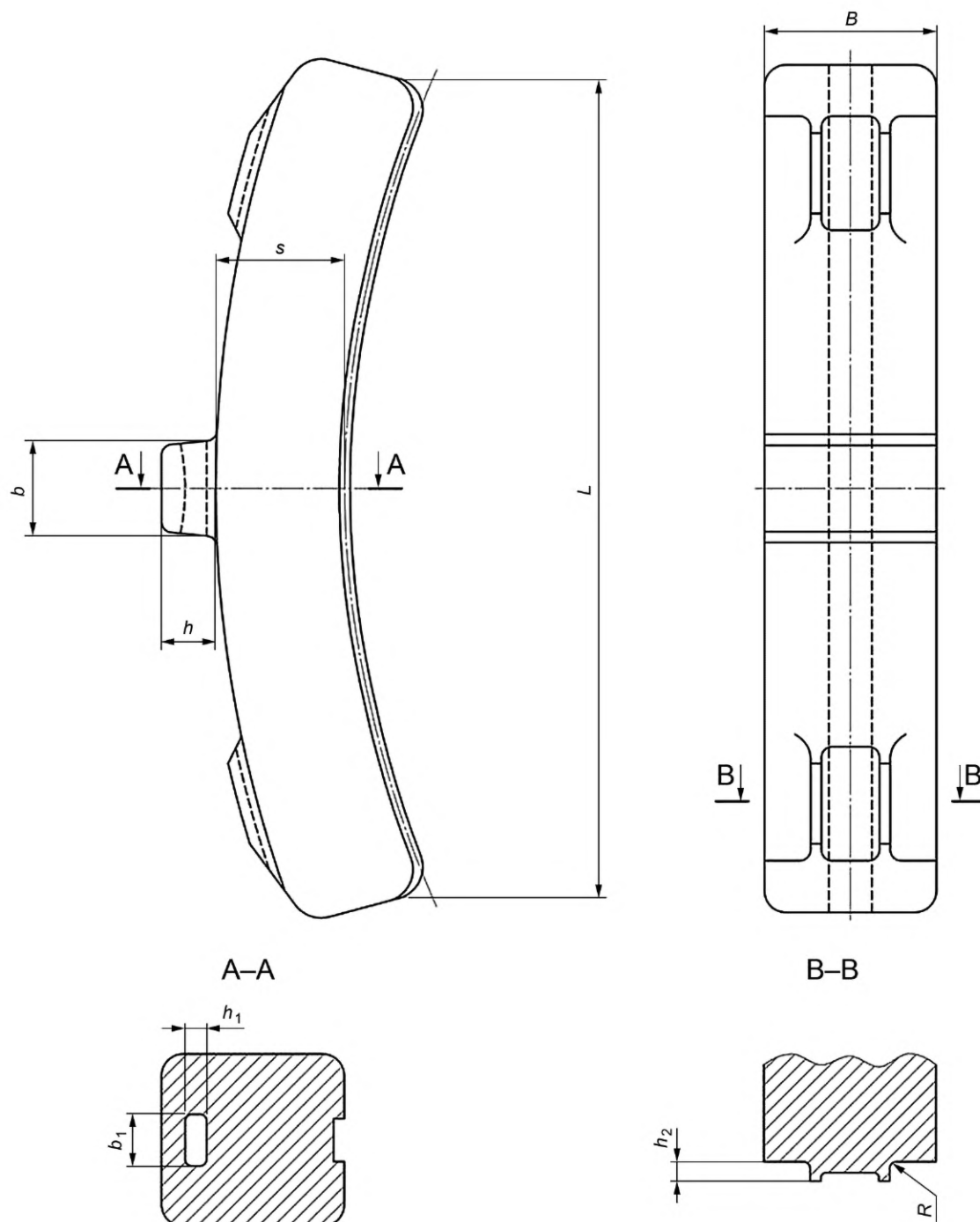
Рисунок А.1 — Тормозная колодка безгребневая чугунная для вагонов (без скобы)
