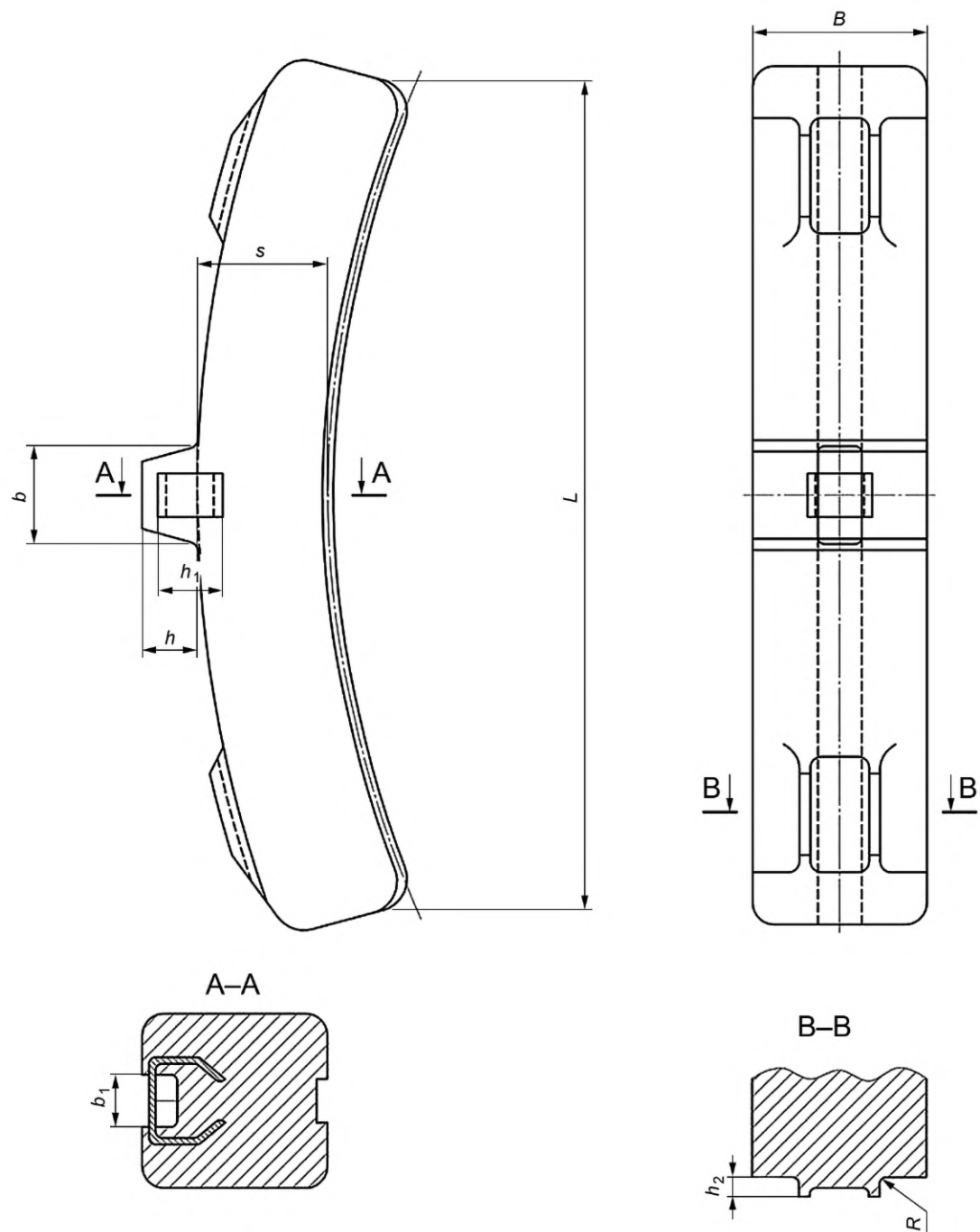
Рисунок А.2 — Тормозная колодка безребневая чугуная для вагонов (со скобой)
