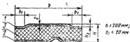
1—наружный лист; 2—внутренний лист; 3—утеплитель
