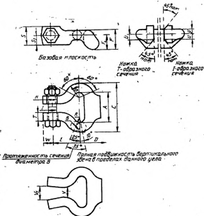
Рисунок 1 — Соединительное звено
