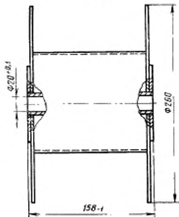
Кассета для намотки кабельных гильз в виде цепи
