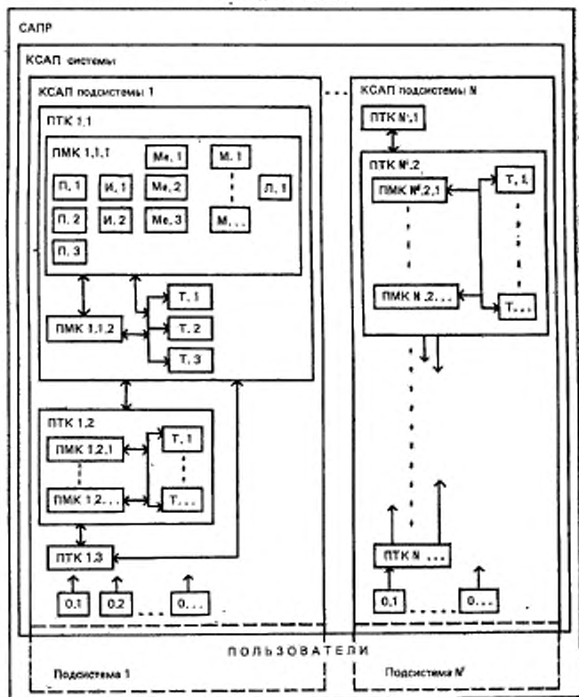
Структурная схема САПР
