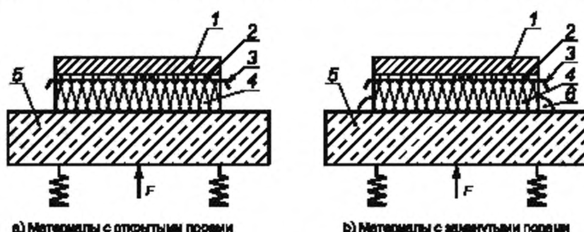
Рисунок Г.1 — Схема возбуждения нагружающей пластины. Измерение вибрации нагружающей пластины
