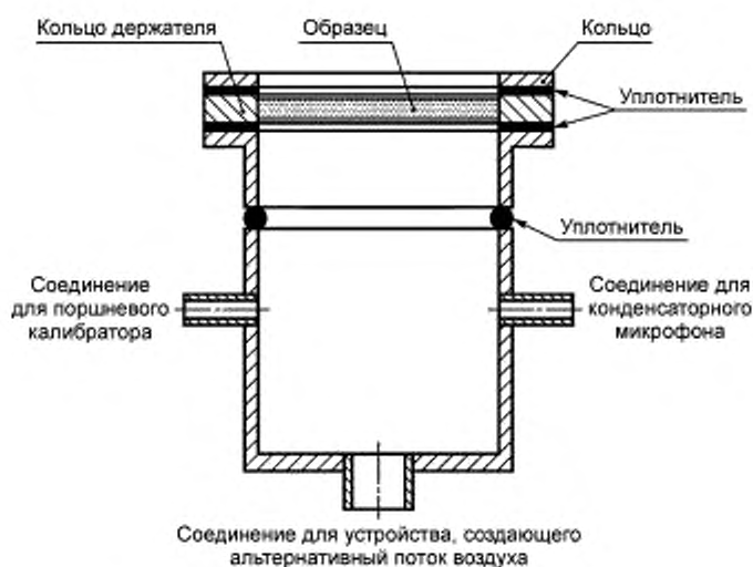
Рисунок Б.5 — Схема измерительной камеры с держателем для цилиндрического образца (метод В)
