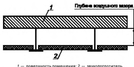
Рисунок В.2 — Схема размещения образцов материала при проведении испытаний
