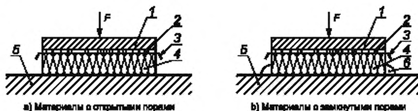
Рисунок Г.1 — Схема возбуждения нагружающей пластины. Измерение вибрации нагружающей пластины
