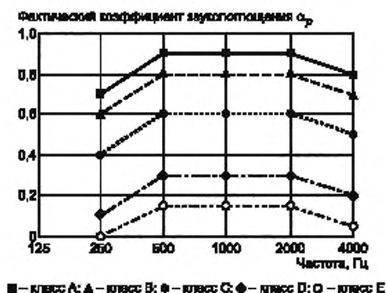
Рисунок 1 — Нормативные кривые, ограничивающие классы звукопоглощения
