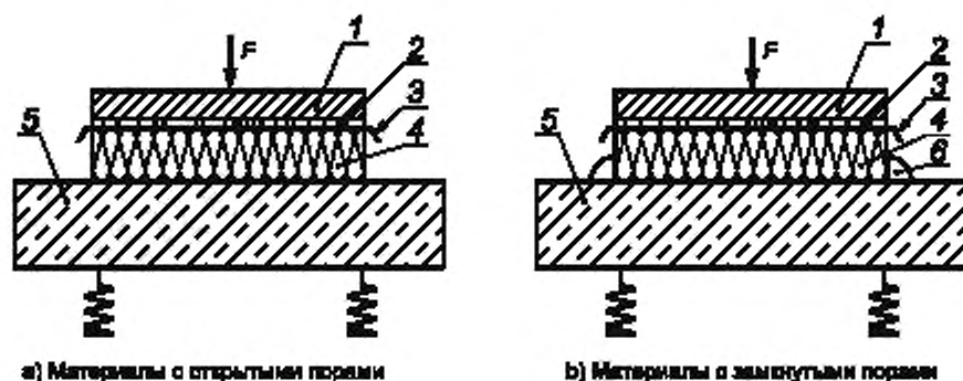
Рисунок Г.2 — Схема возбуждения нагружающей пластины. Измерение вибрации нагружающей пластины и основания
