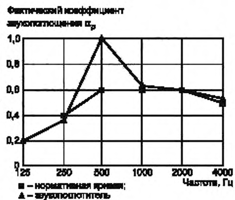
Рисунок В.4 — Пример определения индекса звукопоглощения с применением индикатора формы \alpha_w [\alpha_w = 0,60 (M)]
