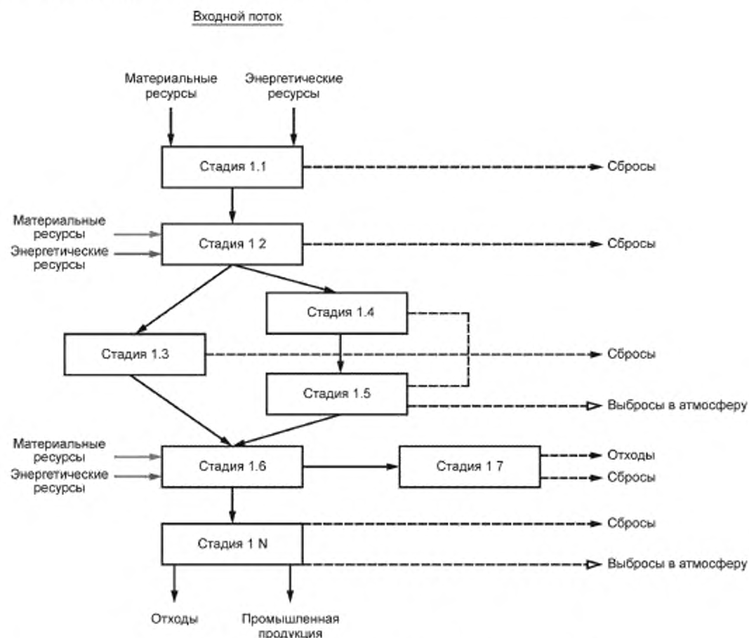
Рисунок 1 — Общая схема описания технологического процесса
