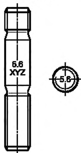
Рисунок 14 — Пример маркировки шпилек
