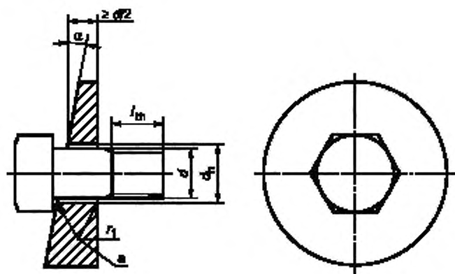
а) Радиус или фаска 45°. См. таблицу 15.
