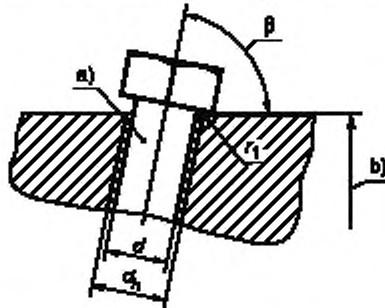
Рисунок 7 — Устройство для испытания головки на прочность
