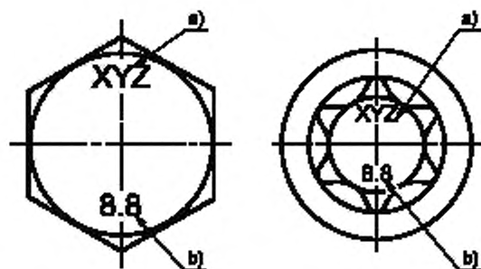
Рисунок 11 — Примеры маркировки болтов и винтов с шестигранной и звездообразными головками
