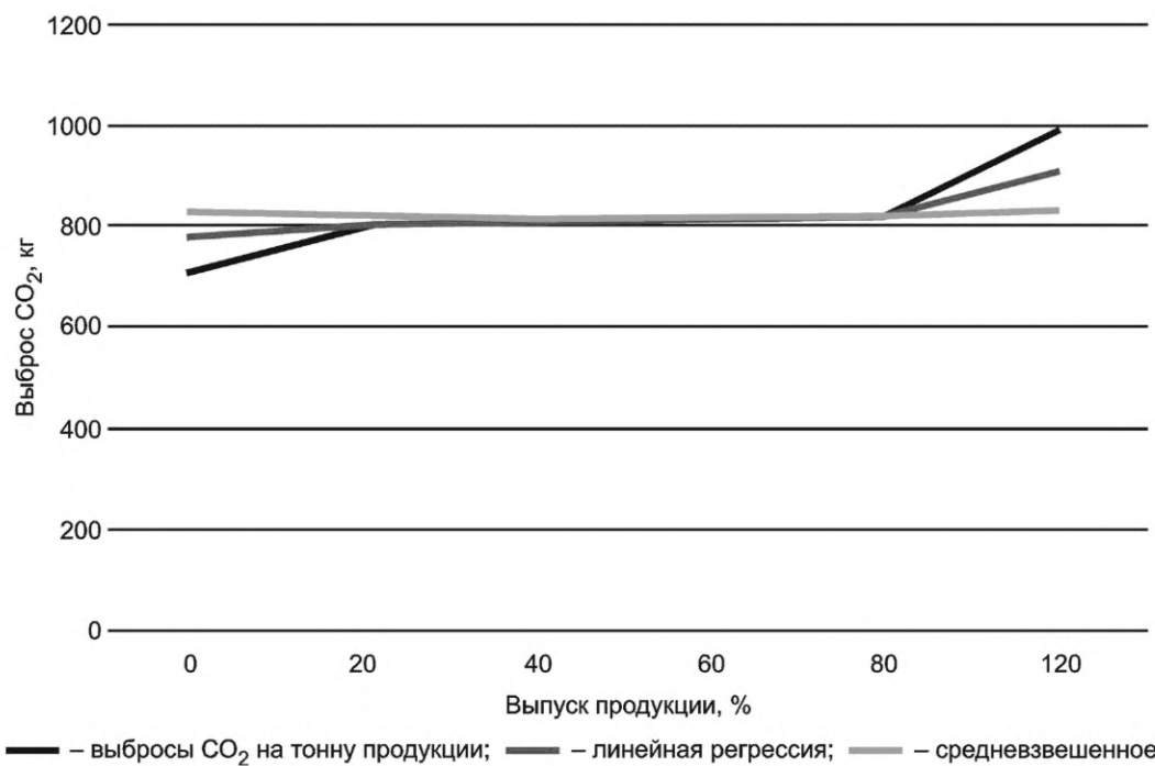
Рисунок В.1 — Пример построения кривых бенчмаркинга удельных выбросов парниковых газов
