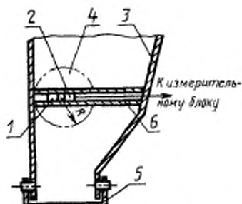
1 — источник излучения; 2 — детектор; 3 — расходный бункер; 4 — сфера зоны рас- сеяния нейтронов; 5 — шпиль; 6 — обсад- ная труба
