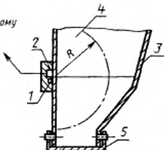
1 — источник излучения; 2 — детектор; 3 — расходный бункер; 4 — полусфера зо- ны рассеяния нейтронов; 5 — шпиль
