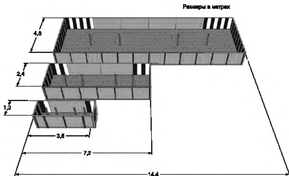
Рисунок 1 — Три типоразмера ограниченных участков, покрытых песком
