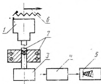
1 — узел опоры ротора с электромагнитным приводом; 2 — матрица с ротором; 3 — нагружающее устройство; 4 — регулятор; 5 — прибор КСП-4; 6 — устройство задатчик амплитуды.
