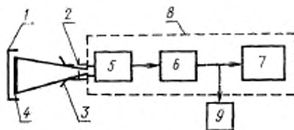
1—световой шкаф; 2—светофильтры; 3—тубус; 4—испытательная таблица; 5—телевизионная камера; 6—приборы в составе ПТУ; 7—видеоконтрольное устройство; 8—ПТУ; 9—осциллограф
