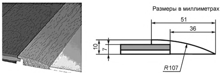
Рисунок А.3 — Иллюстрация установки деревянной планки
