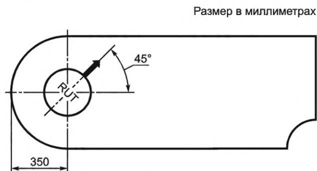
Рисунок 5 — Исходная позиция робота для преодоления одиночной ступени
