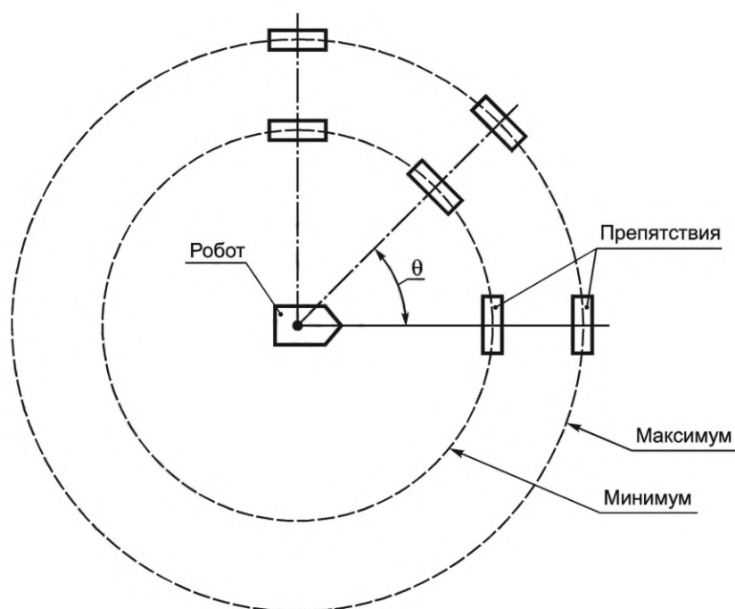
Рисунок 7 — Компоновка испытательного стенда для обнаружения препятствий
