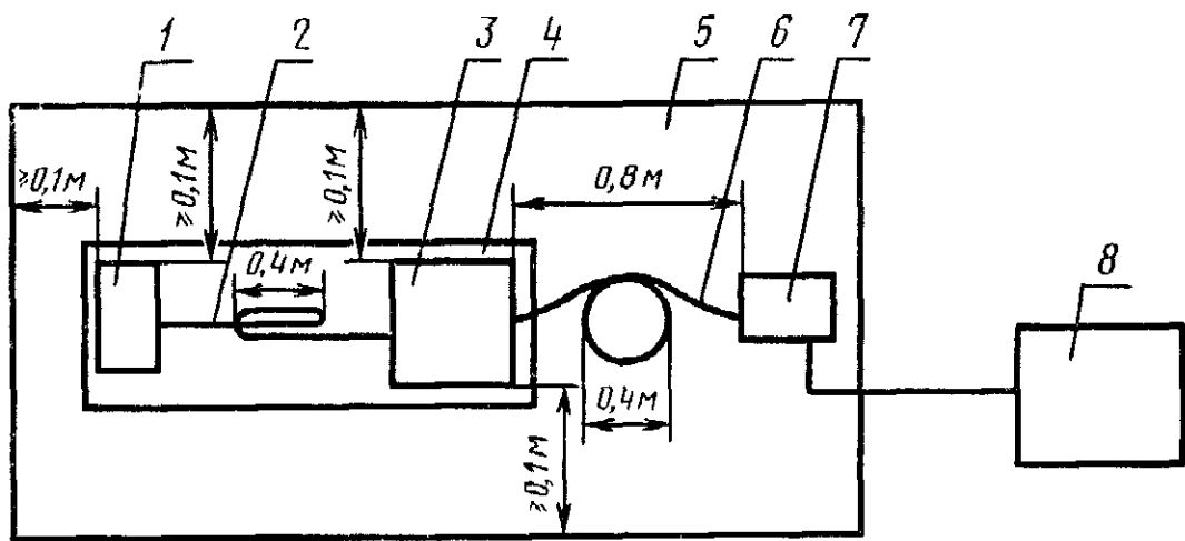
1—внешнее устройство; 2—кабель для подключения внешних устройств; 3—испытуемая установка; 4—подставка из изоляционного материала; 5—металлический лист; 6—кабель для подключения к сети электропитания; 7—эквивалент сети; 8—измеритель радиопомех
