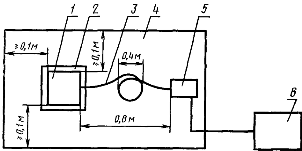
1—испытуемая установка; 2—подставка из изоляционного материала; 3—кабель для подключения установки к сети электропитания; 4—металлический лист; 5—эквивалент сети; 6—измеритель радиопомех
