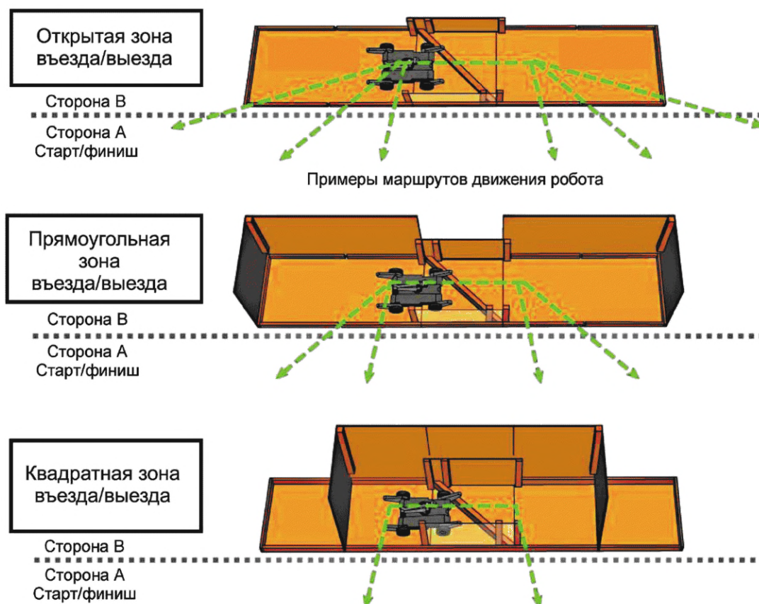
Рисунок 2 — Испытательный стенд с открытой, прямоугольной и квадратной зонами въезда/выезда и примерами маршрутов движения робота
