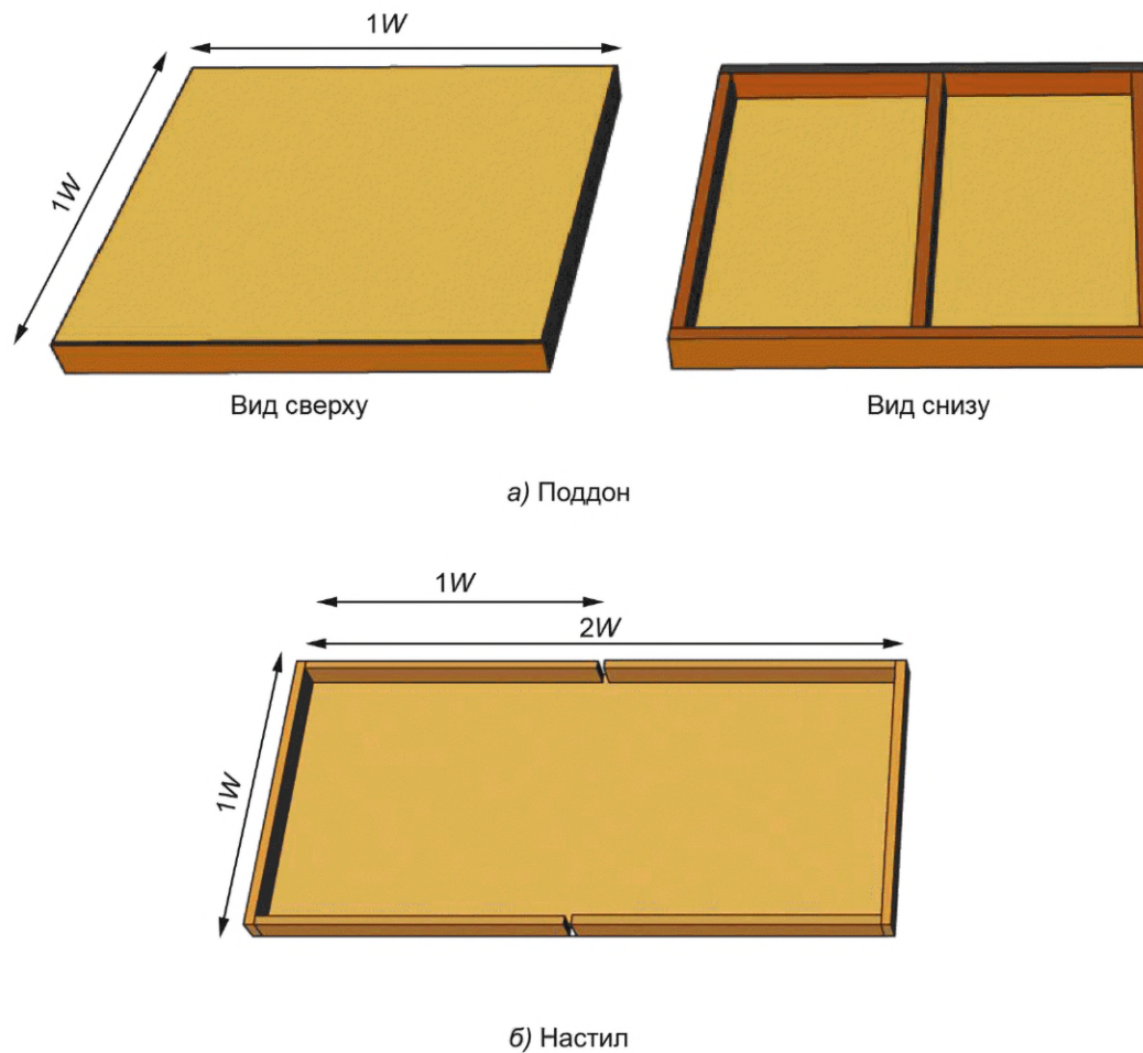
Рисунок 6 — Поддон и настил
