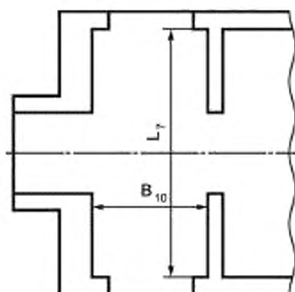
Рисунок 16 — Тамбур
