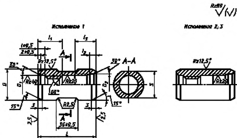
Рисунок 4 — Переводная муфта
