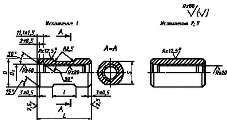
Рисунок 3 — Соединительная муфта
