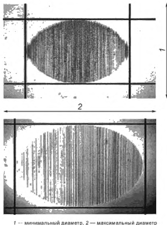
Рисунок 2 — Типичные пятна износа и определение размера
