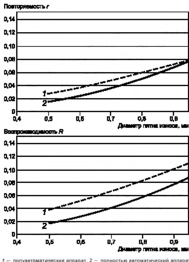
Рисунок 4 — Прецизионность метода
