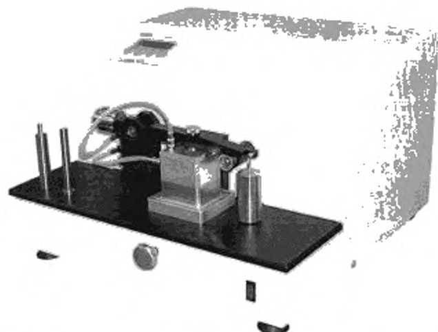
Рисунок А2.1 — Полностью автоматический аппарат для оценки смазывающей способности в системе «шар-цилиндр»
